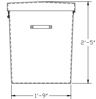
RIGHT ELEVATION
